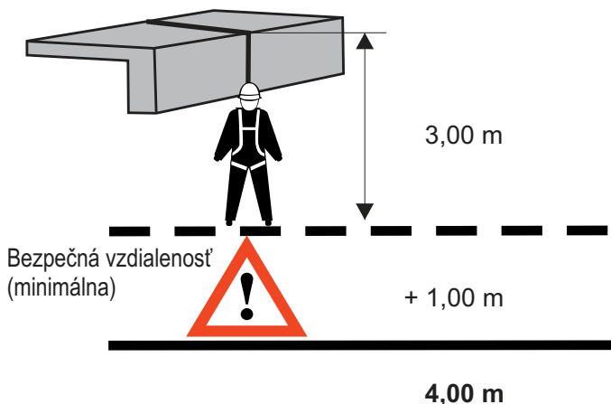
Obr. 15 Pravouhlý pád cez hranu
