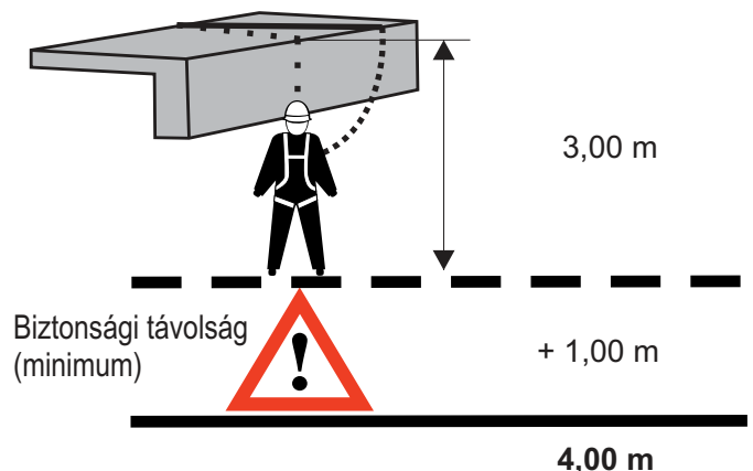
16. kép Oldalirányú zuhanás peremen keresztül
