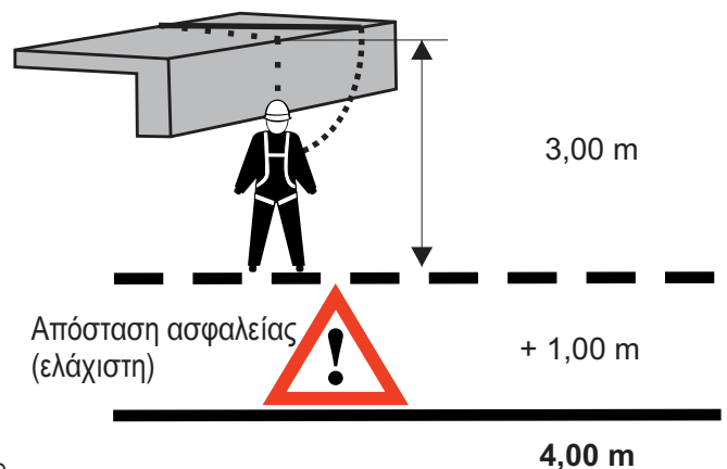
Εικόνα 16 Πλευρική πτώση μέσω ακμών
