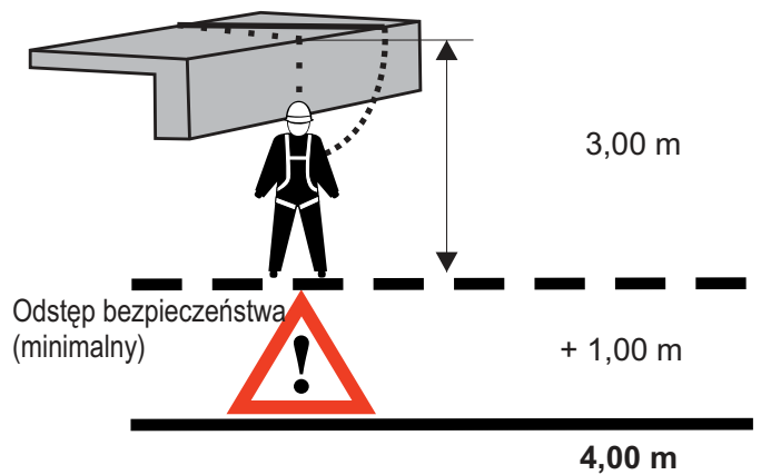
Zdjęcie 16 Upadek boczny przez krawędź
