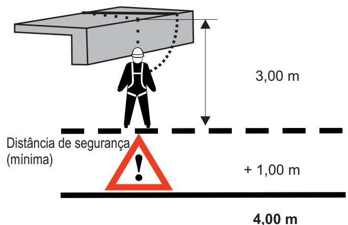
Figura 16 queda lateral sobre arestas
