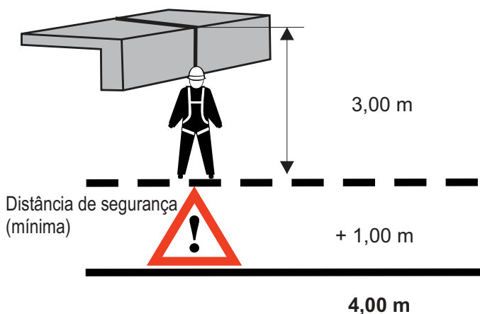
Figura 15 queda em ângulo recto sobre arestas
