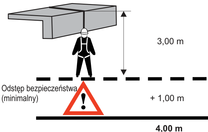
Zdjęcie 15 Upadek przez krawędź pod kątem prostym
