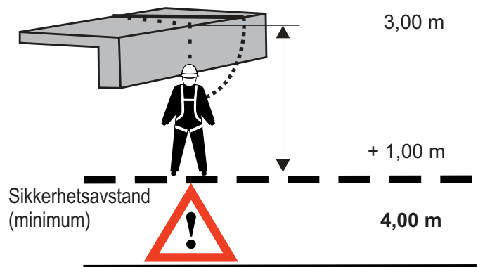
Bilde 16 Sideveis fall over kant
