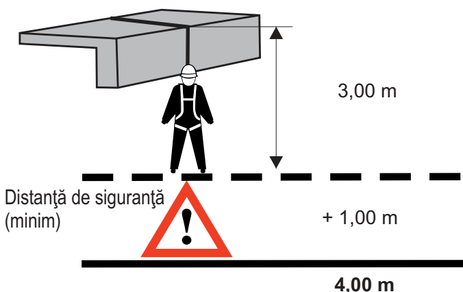
Imaginea 15 Cădere în unghi drept peste muchii
