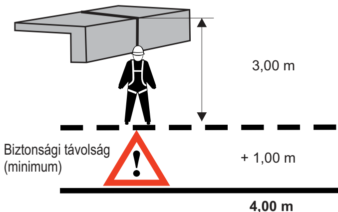
15. kép Merőleges irányú zuhanás peremen keresztül
