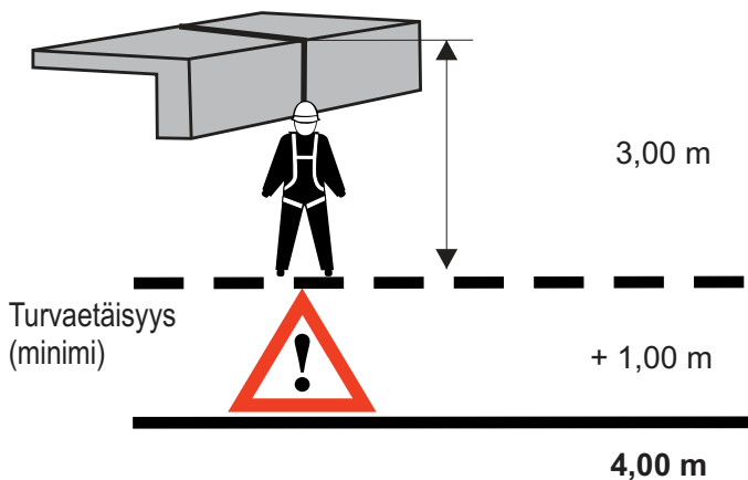
Kuva 15 suorakulmainen putoaminen reunojen yli
