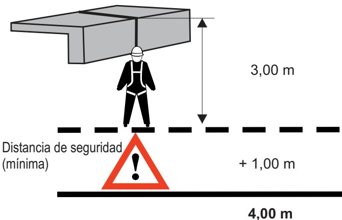
Imagen 15 Caída en ángulo recto por bordes
