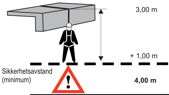
Bilde 15 Rettvinklet fall over kant
