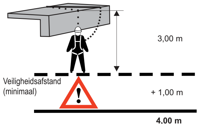
Afbeelding 16 Val zijdelings omlaag over kanten of randen
