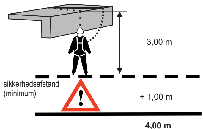
Figur 16 sidelæns fald over kanter
