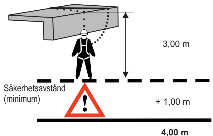
Bild 16 Sidofall över kanten
