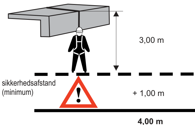
Figur 15 fald over kanter i en ret vinkel
