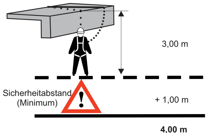
Bild 16 seitlicher Sturz über Kanten
