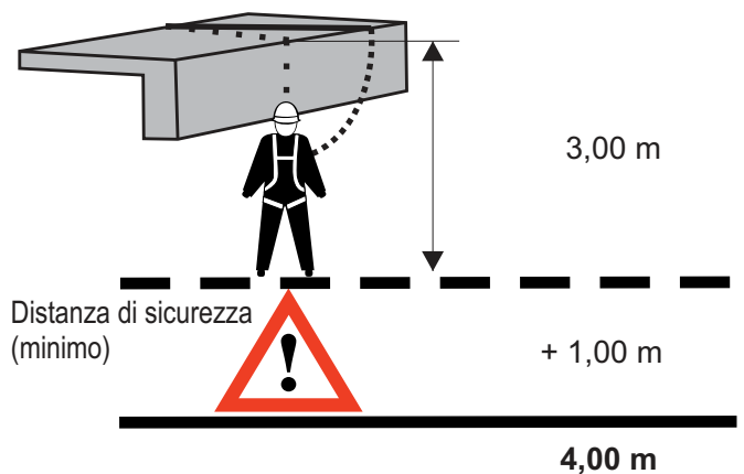
Immagine 16 Caduta laterale rispetto allo spigolo
