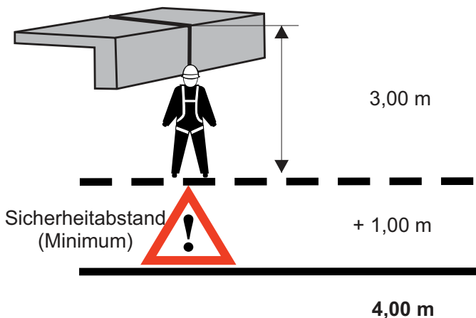
Bild 15 rechtwinkliger Sturz über Kanten
