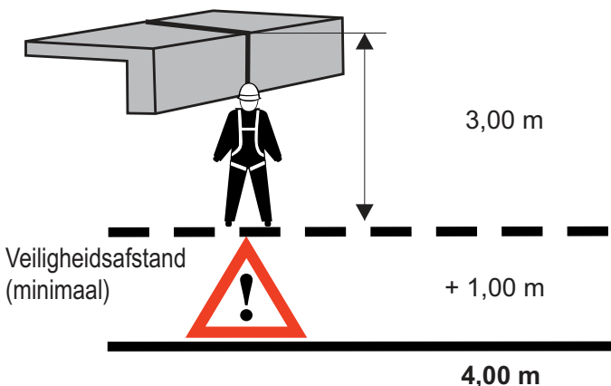
Afbeelding 15 Val haaks omlaag over kanten of randen
