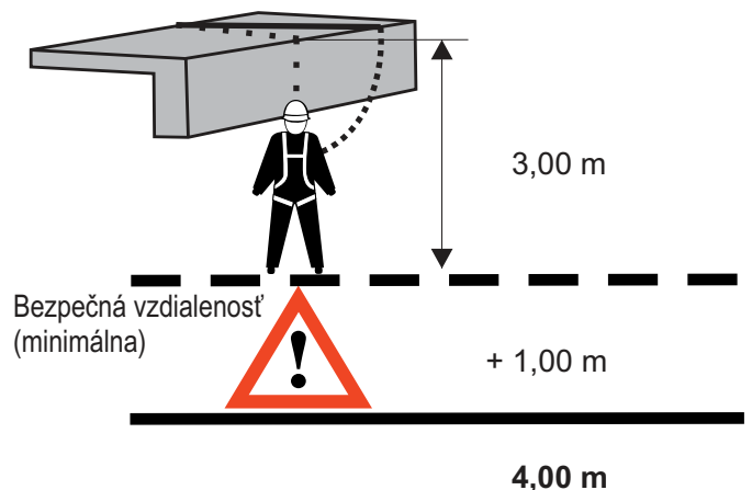
Obr. 16 Bočný pád cez hranu
