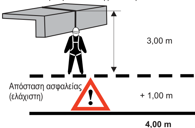
Εικόνα 15 Ορθογώνια πτώση μέσω ακμών
