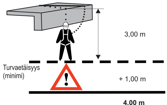
Kuva 16 sivuttainen putoaminen reunojen yli
