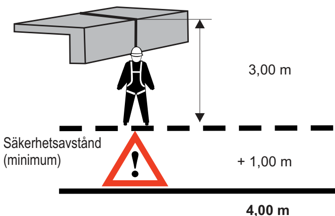
Bild 15 Rätvinkligt fall över kanten
