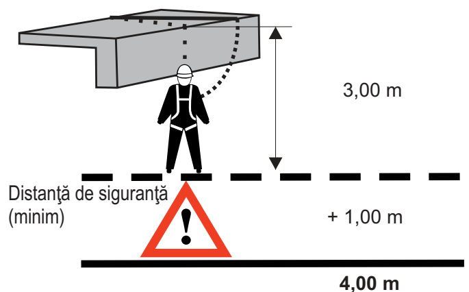
Imaginea 16 Cădere laterală peste muchii
